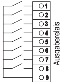
Ausgabereleais
