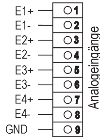
Analogeingänge
