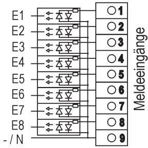
Meldeeingänge
